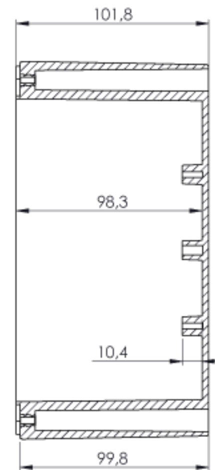
KESIT A-A
