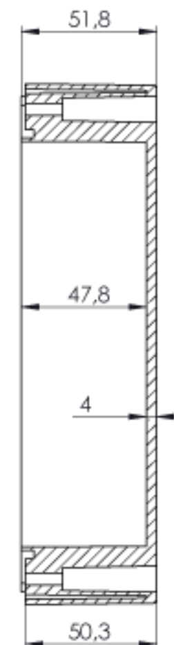
KESIT A-A
