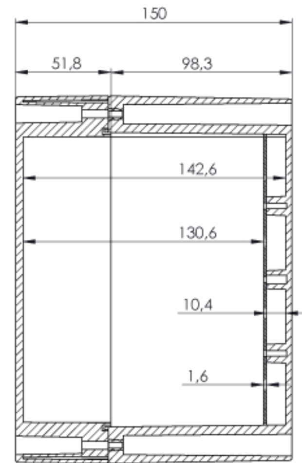
KESIT A-A ÖLÇEK: 1/2
