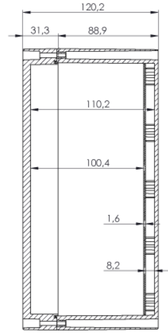
KESIT A-A ÖLÇEK: 1/2
