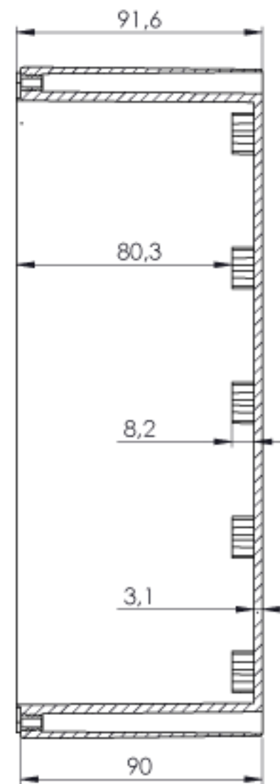
KESIT A-A ÖLÇEK: 1/2
