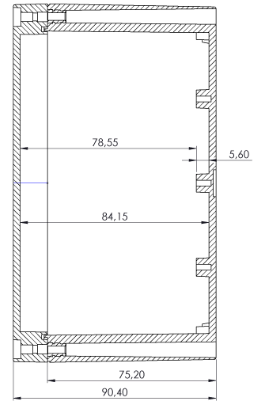
KESIT A-A
