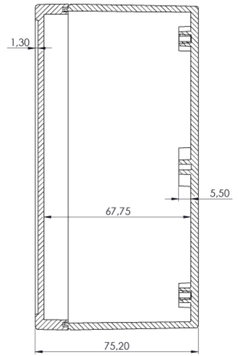
KESIT A-A
