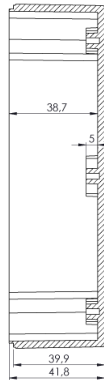
KESIT A-A
