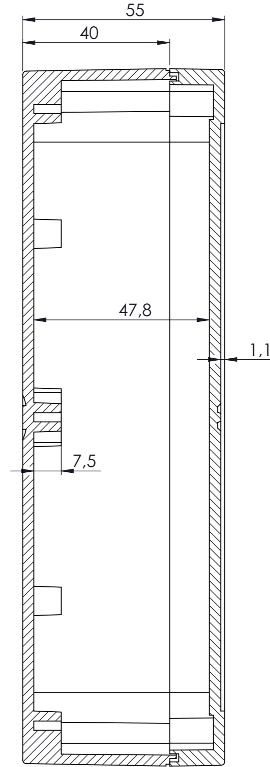
KESIT A-A
