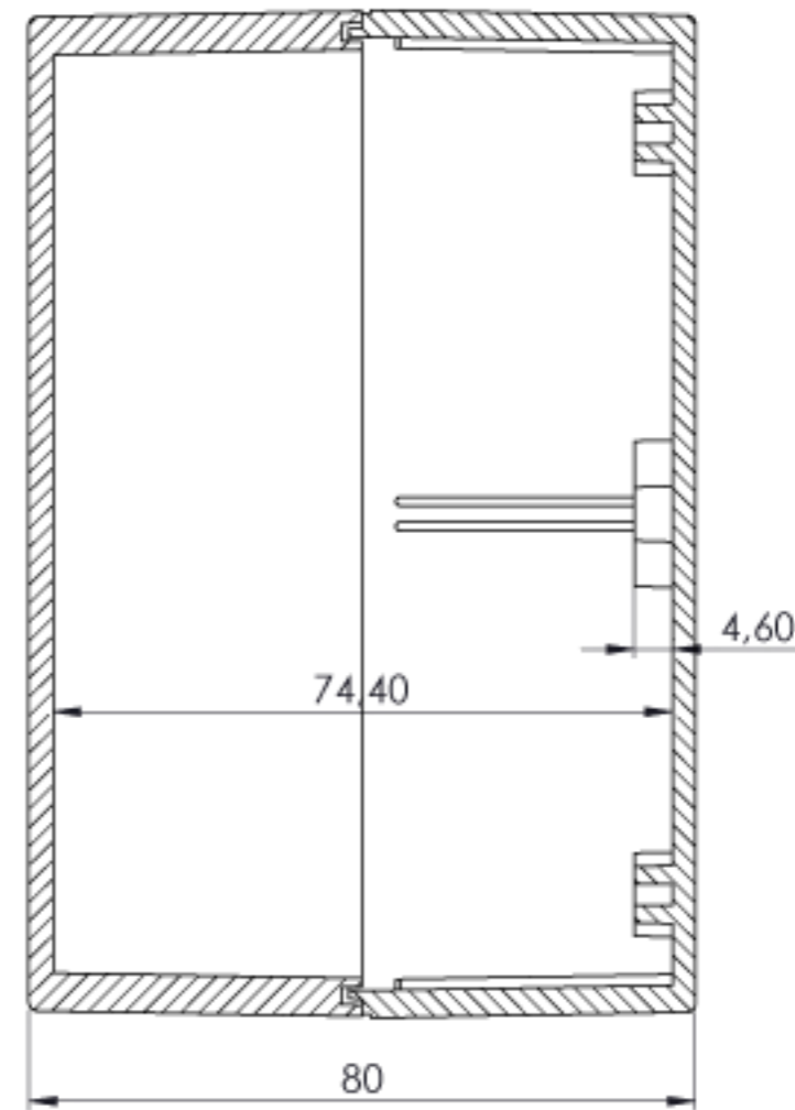
KESIT A-A
