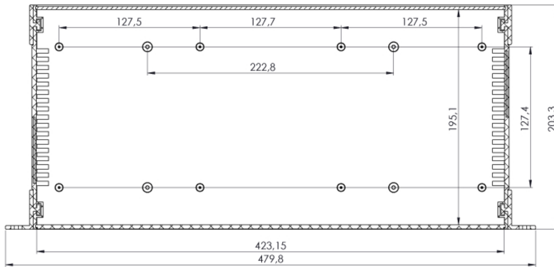
KESIT A-A
