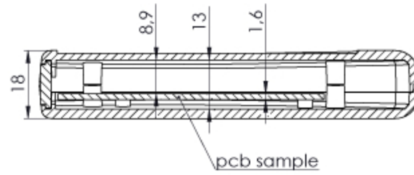
KESIT A-A
