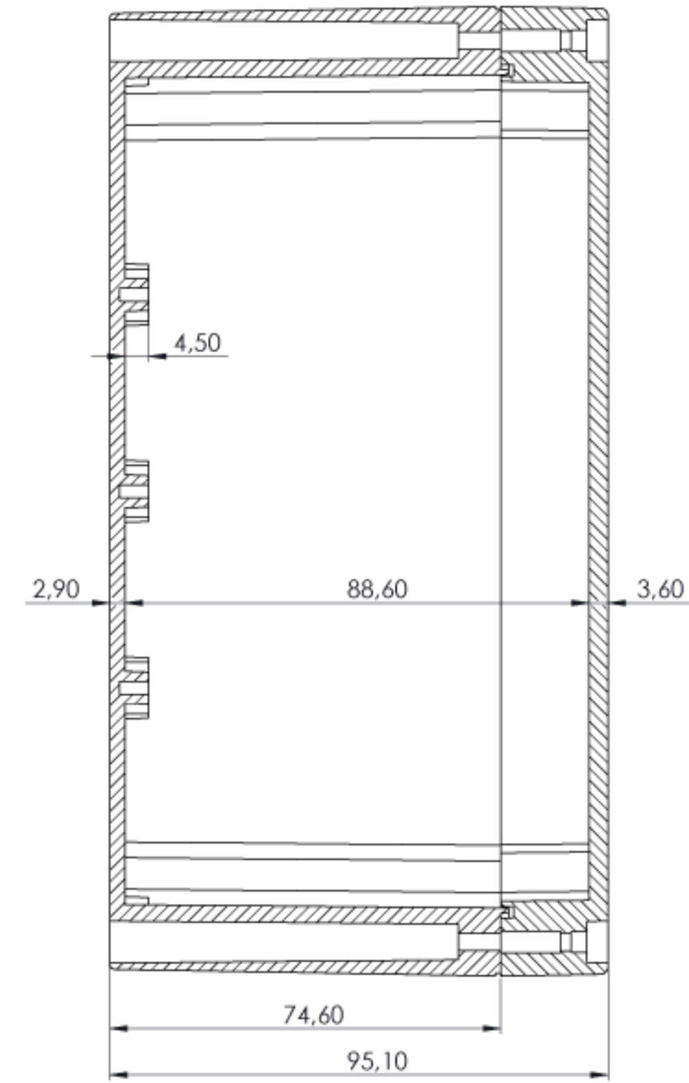
KESIT A-A
