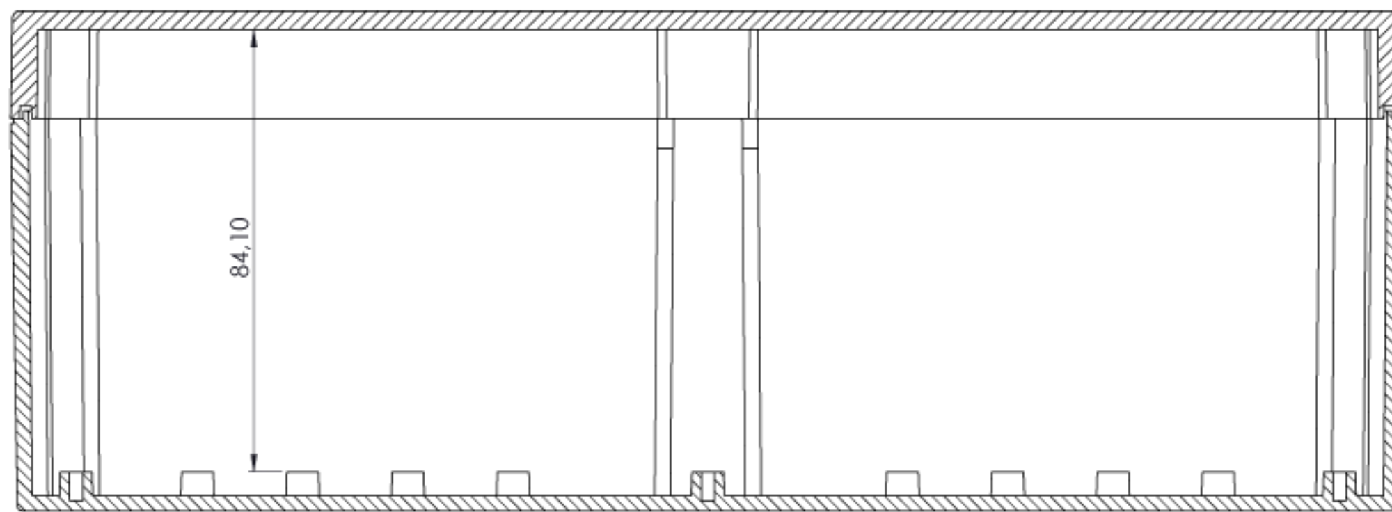
KESIT B-B
