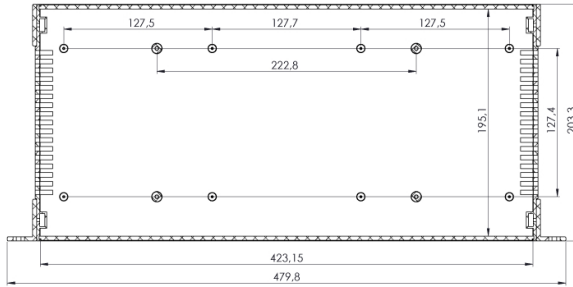
KESIT A-A
