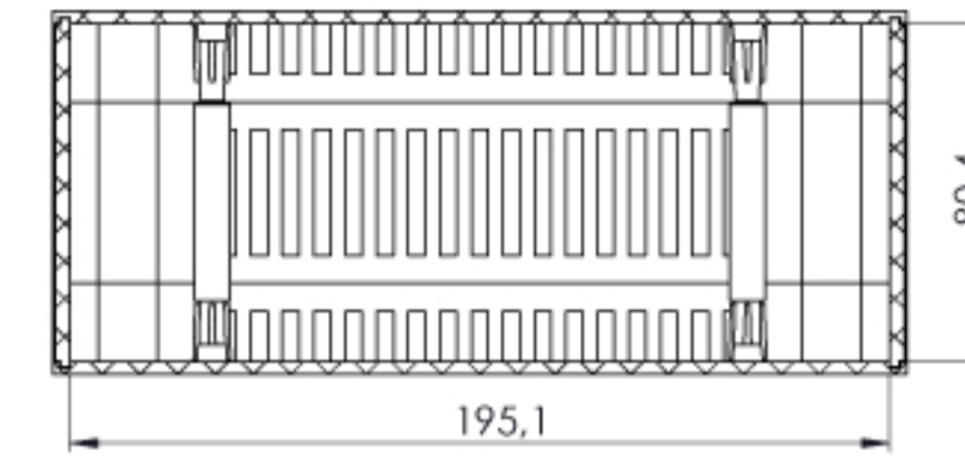
KESIT B-B
