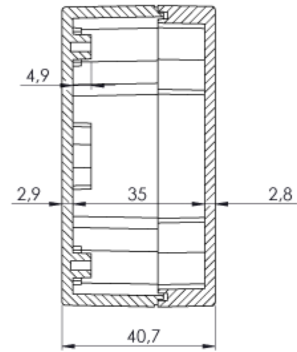
KESIT A-A
